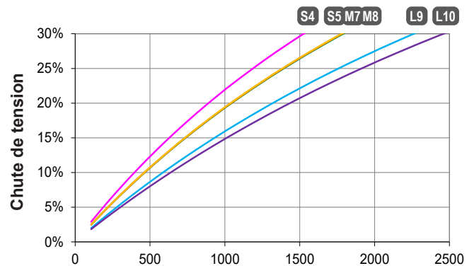
Démarrage des moteurs (AREP/PMG) kVA rotor bloqué à Cos \Phi 0.6
